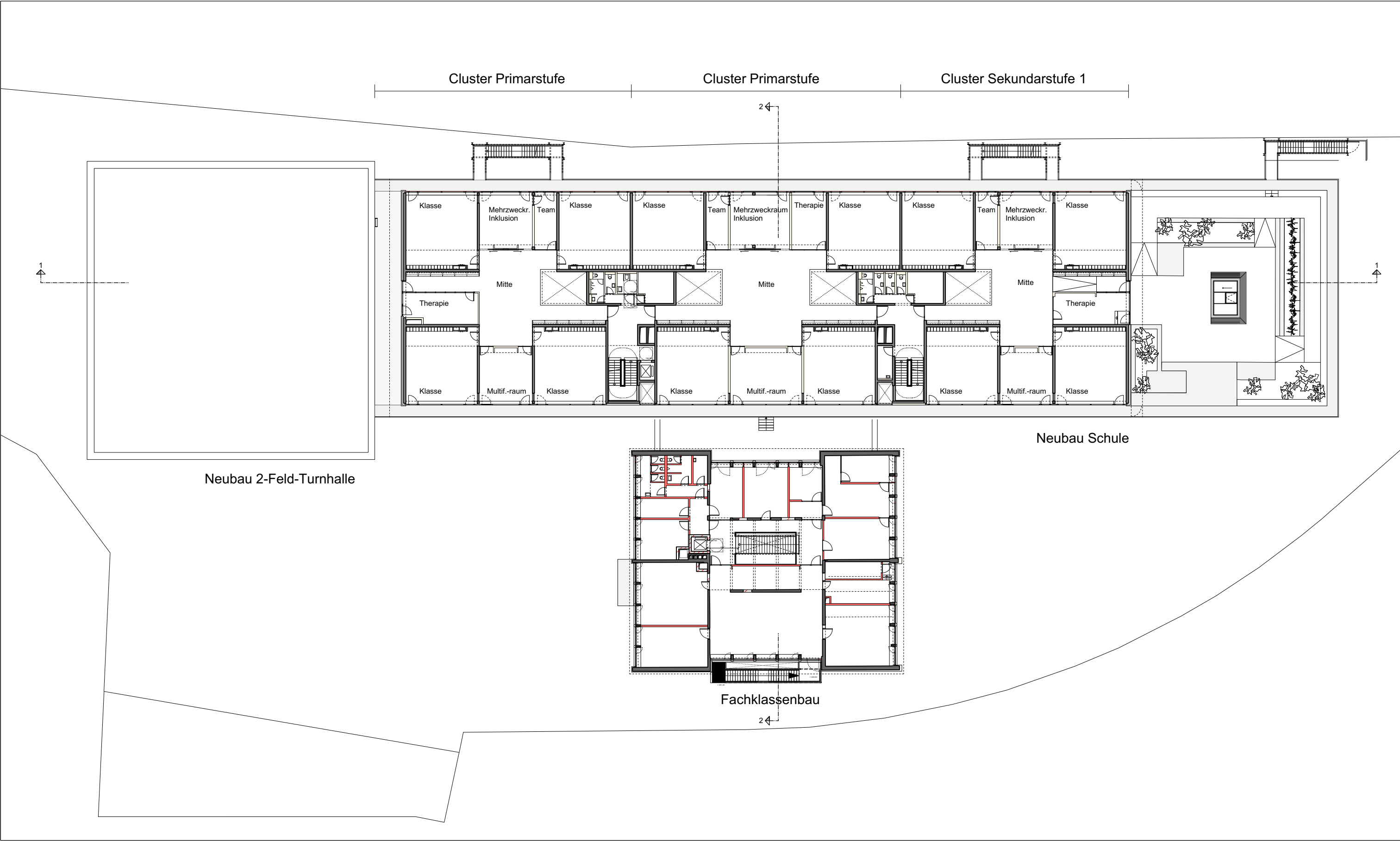
Grundriss 1. Obergeschoss
