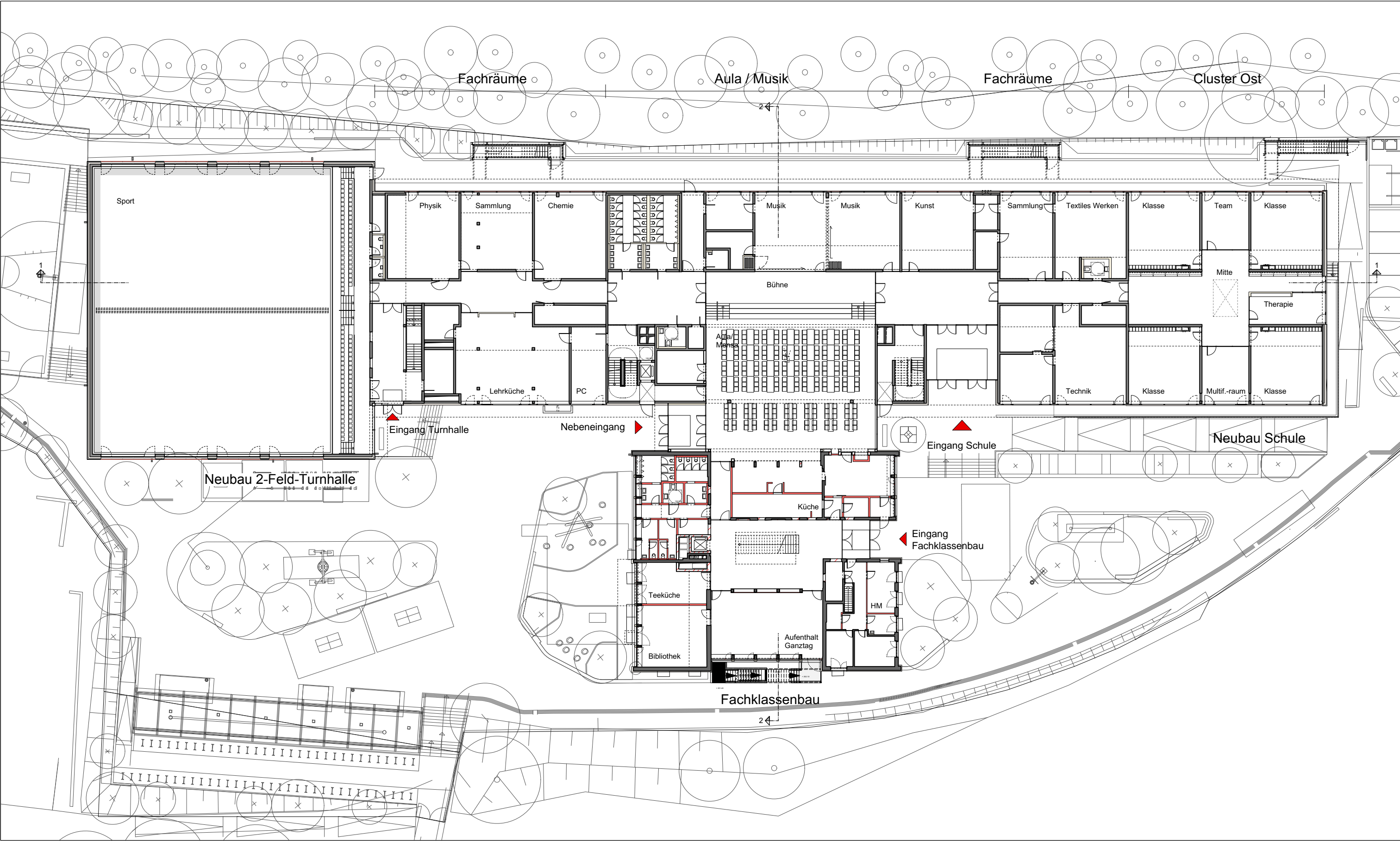
Grundriss Erdgeschoss
