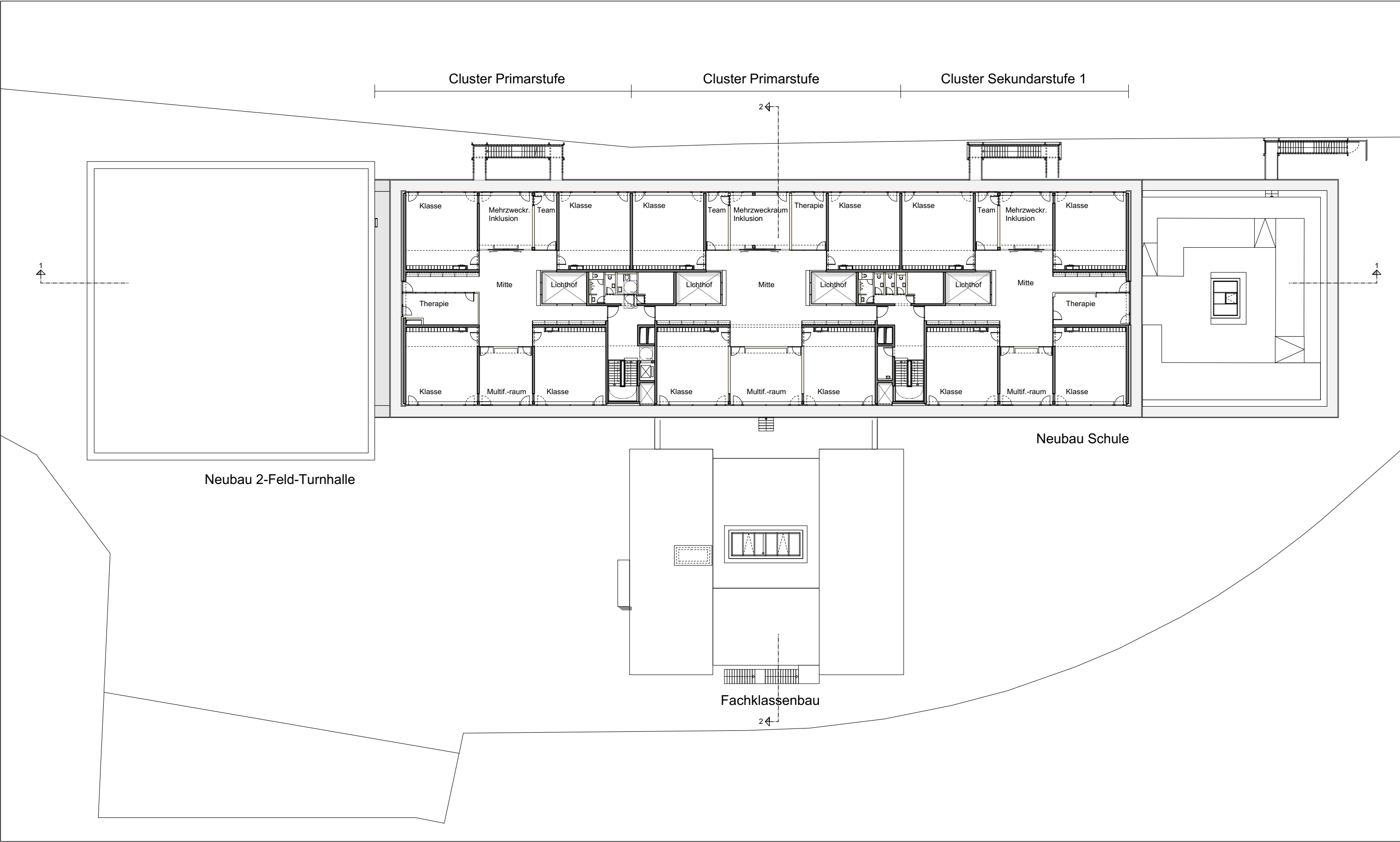
Grundriss 2. Obergeschoss
