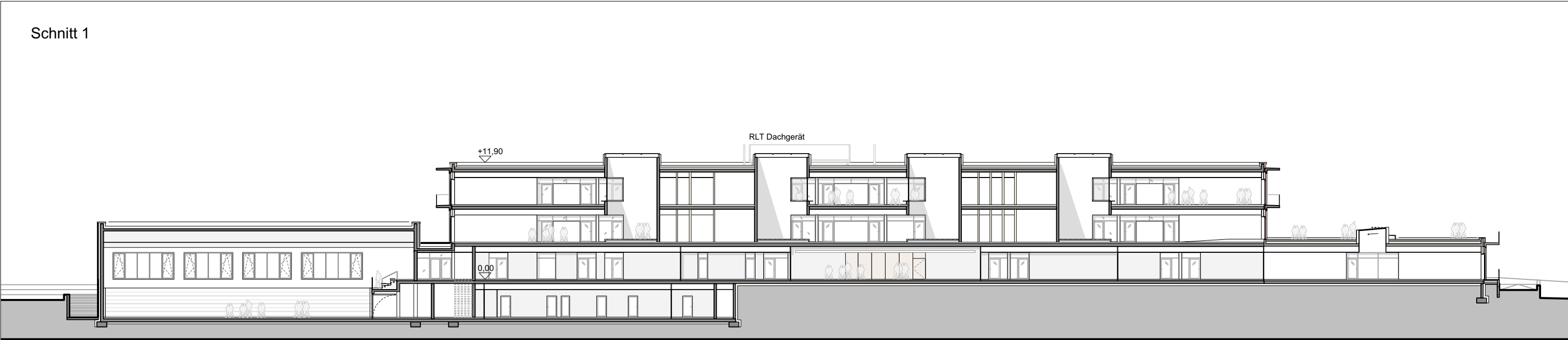
Neubau 2-Feld-Turnhalle
