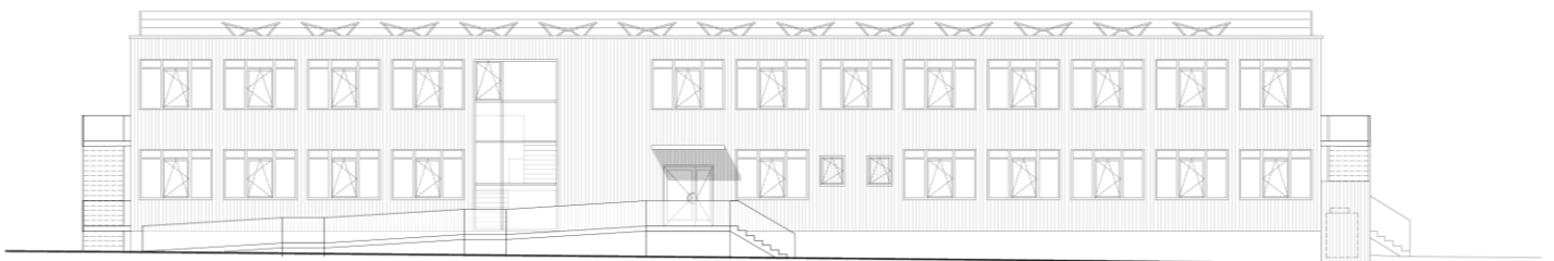
Ansicht Süd
