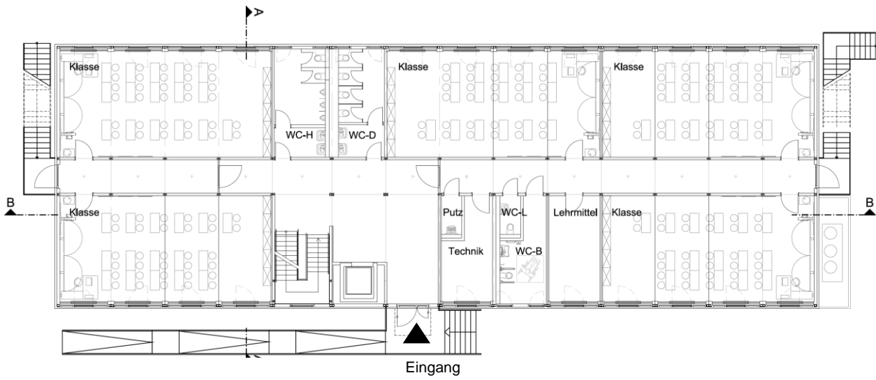
Grundriss Erdgeschoss
