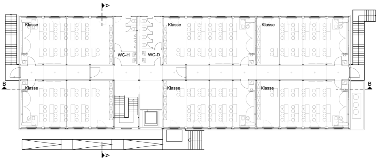
Grundriss Obergeschoss
