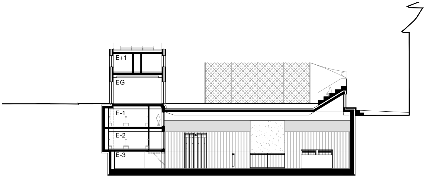
Schnitt A-A | Bau S
