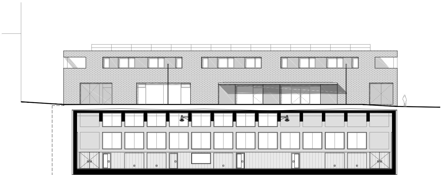
Schnitt B-B | Bau S
