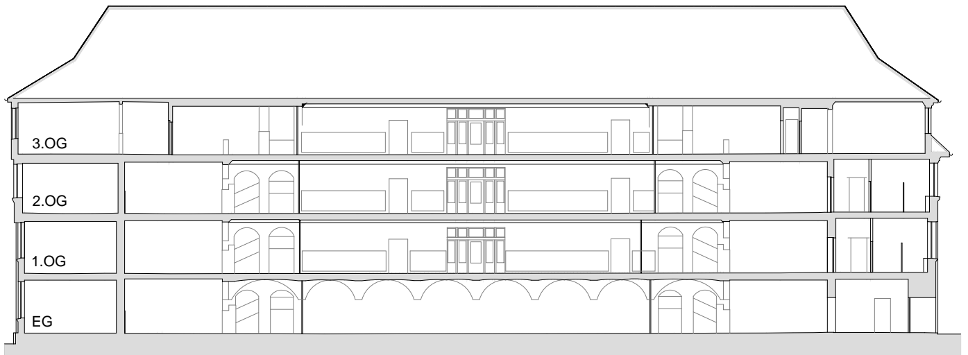
Schnitt B-B | Bau A
