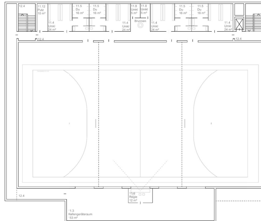
2. Untergeschoss
