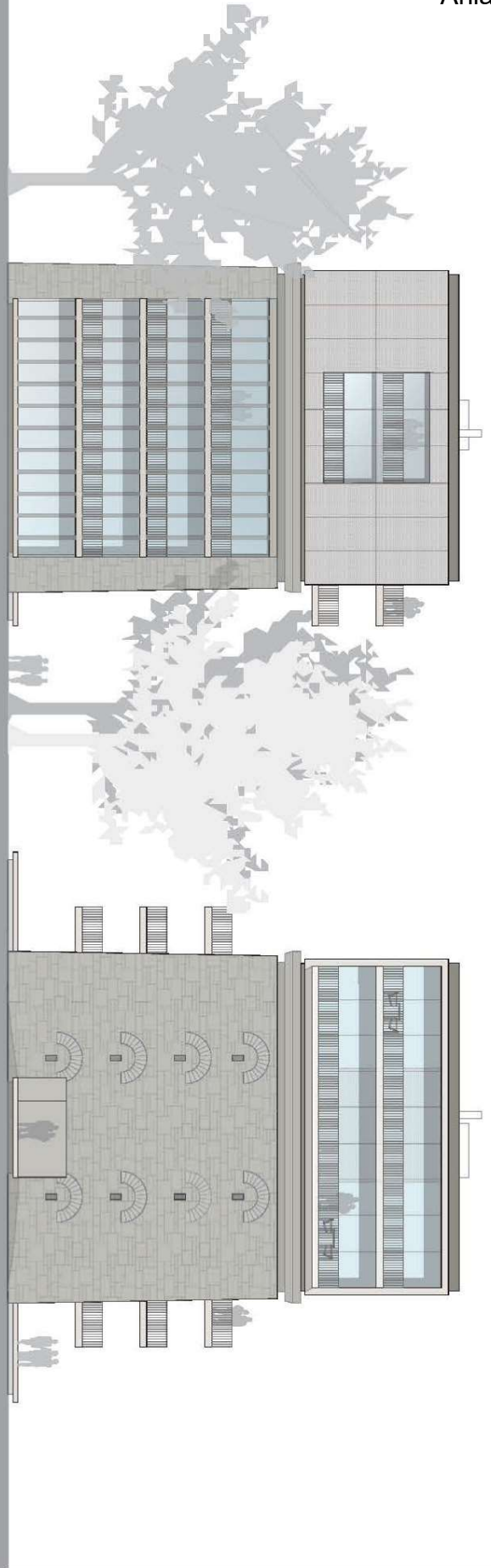
Ansicht West
