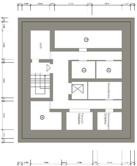
Grundrisse UG 2 M 1:100
