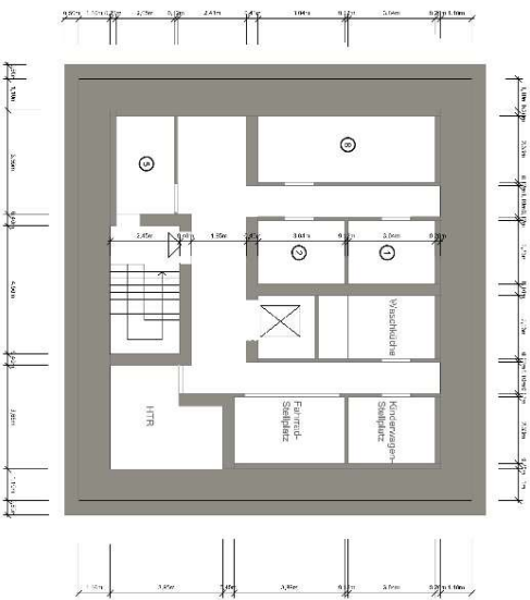
Grundrisse UG 1 M 1:100
