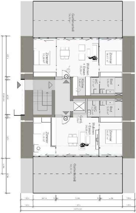
Grundriss EG M 1:100
