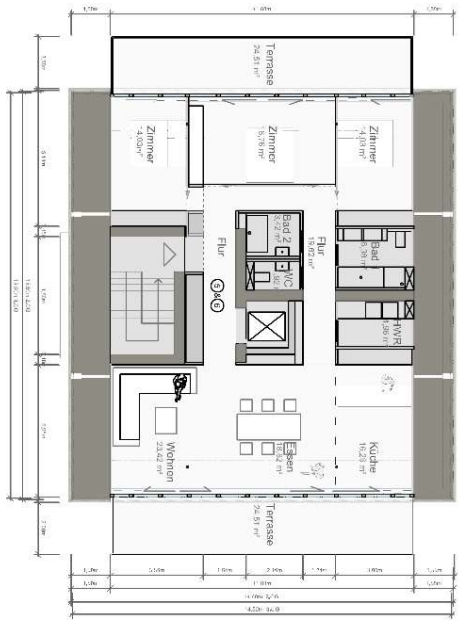
Grundriss OG 2,3 M 1:100
