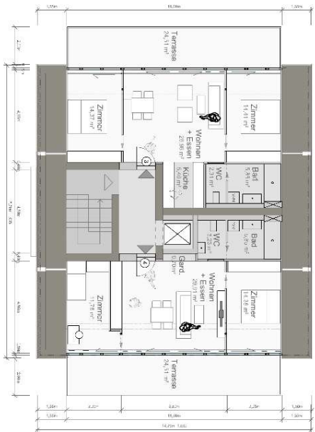
Grundriss 1 OG M 1:100
