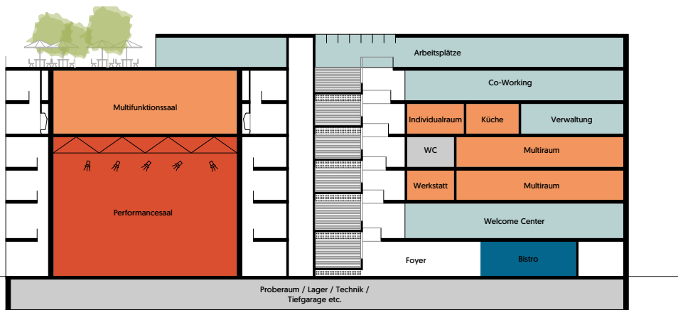
Schnitt B-B
