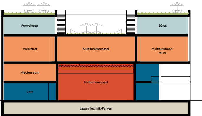
Schnitt A-A
