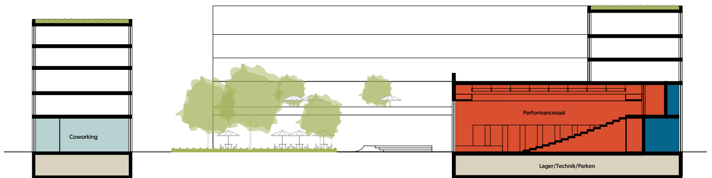
Schnitt B-B
