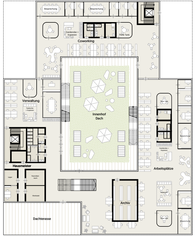
Grundriss 3.OG
