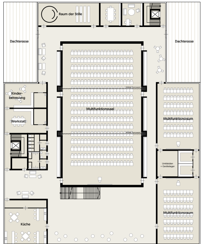
Grundriss 2.OG
