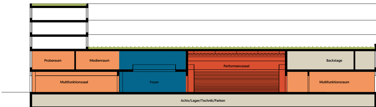
Schnitt A-A
