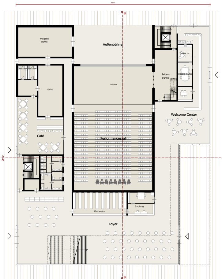
Grundriss EG
