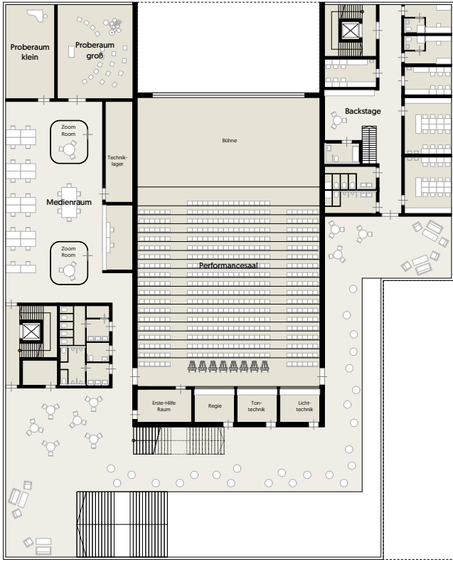
Grundriss 1.OG
