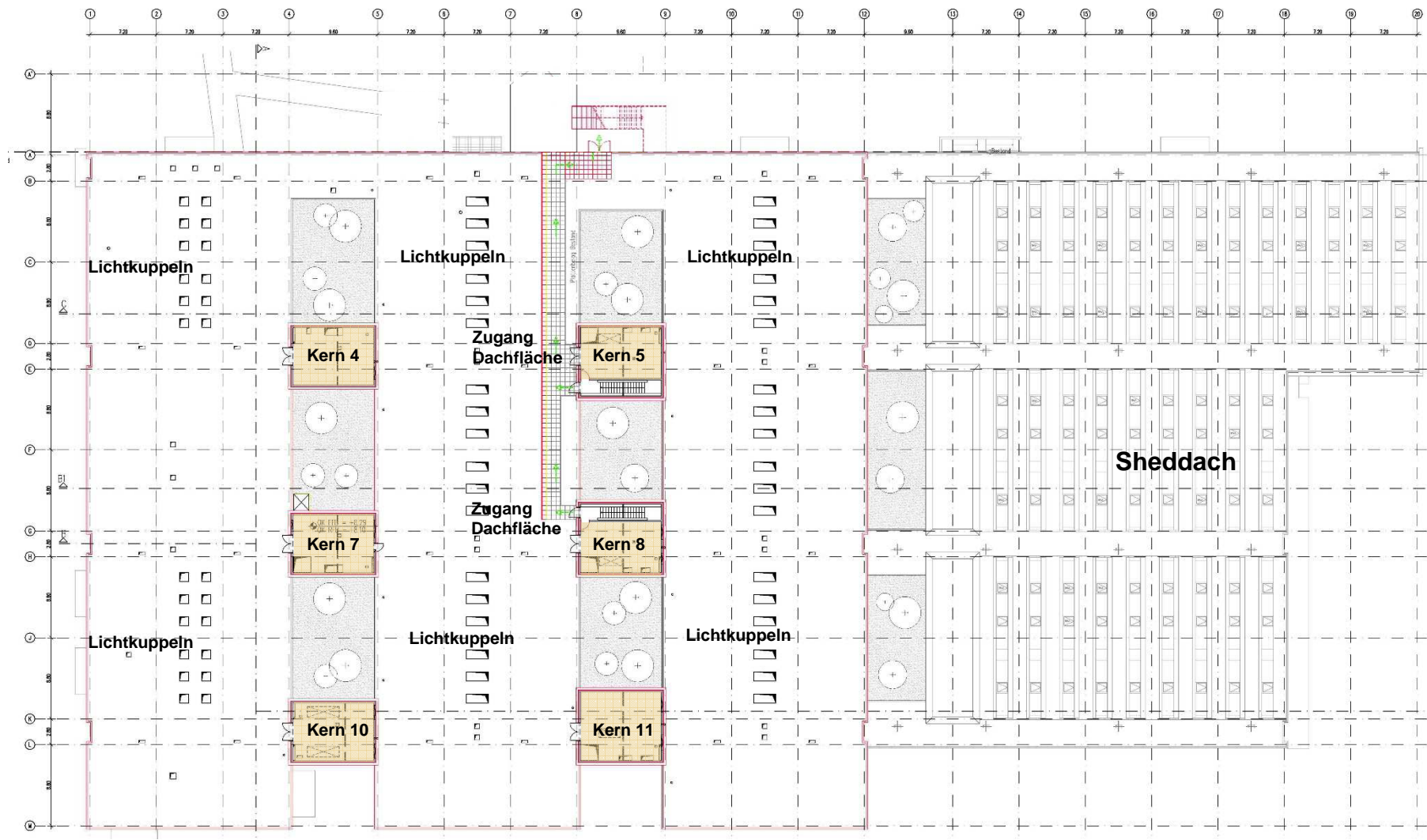
Grundriss 2.OG
