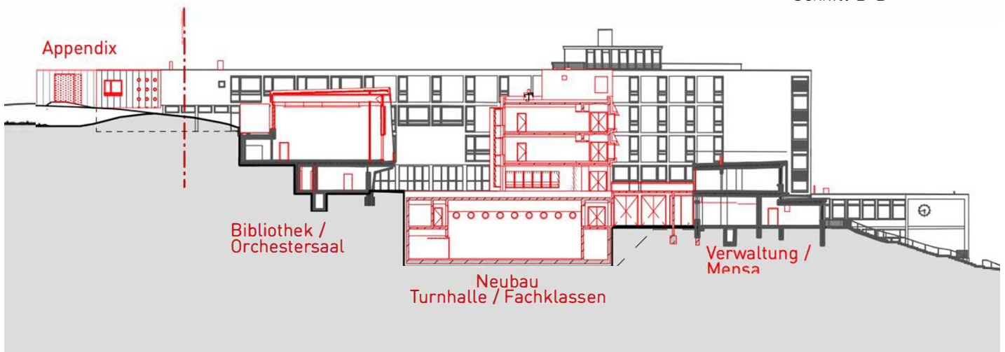
Schnitt A-A
