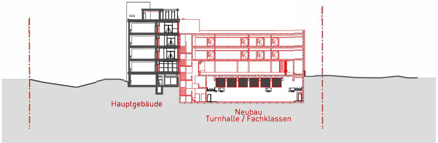
Schnitt B-B
