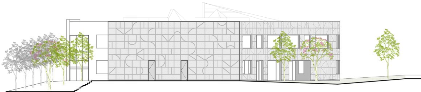
ANSICHT WEST
