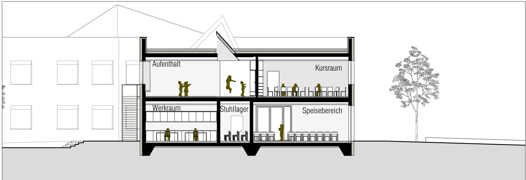
SCHNITT G-G'
