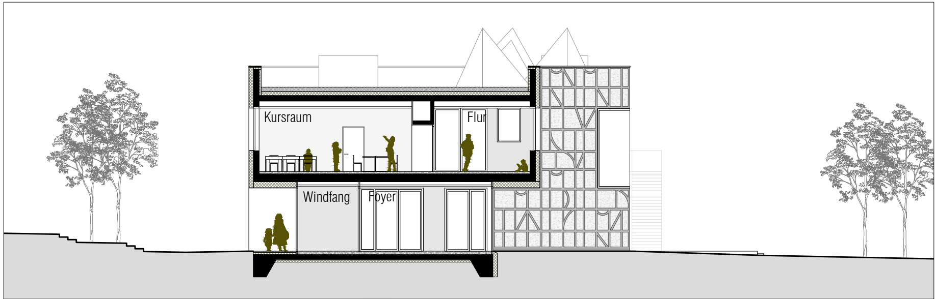
SCHNITT I-I'
