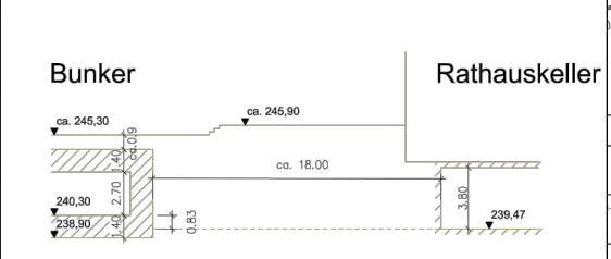
Schnitt B-B
