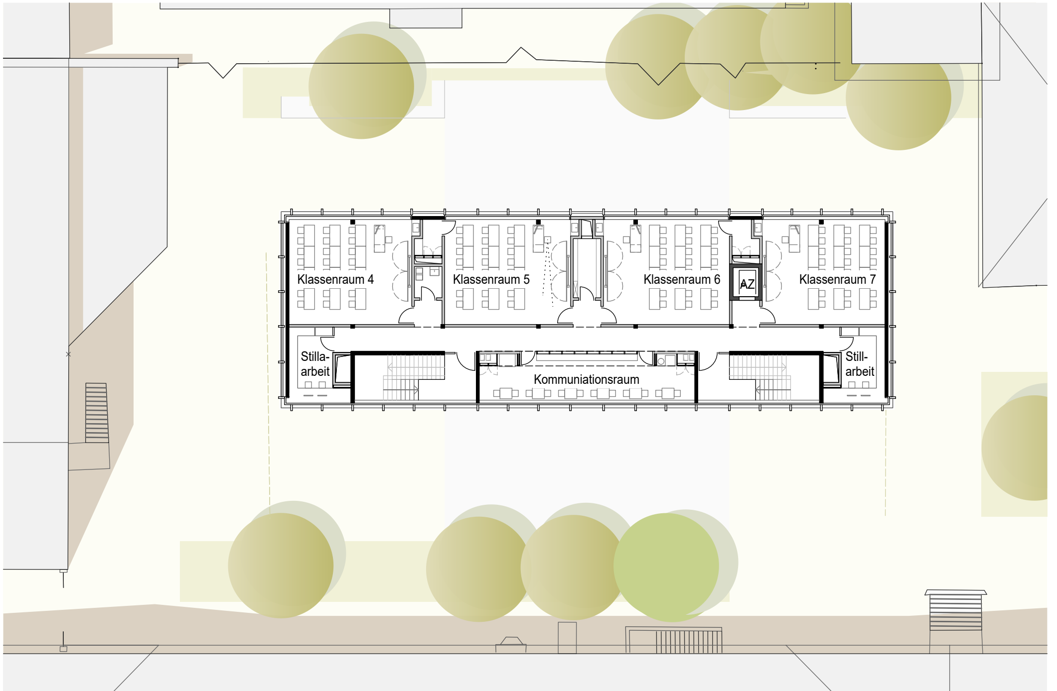
D'Inka Scheible Hoffmann Architekten BDA - Entwurf Mensa und Erweiterung Zeppelin-Gymnasium, Stuttgart Ost - Grundriss OG2
