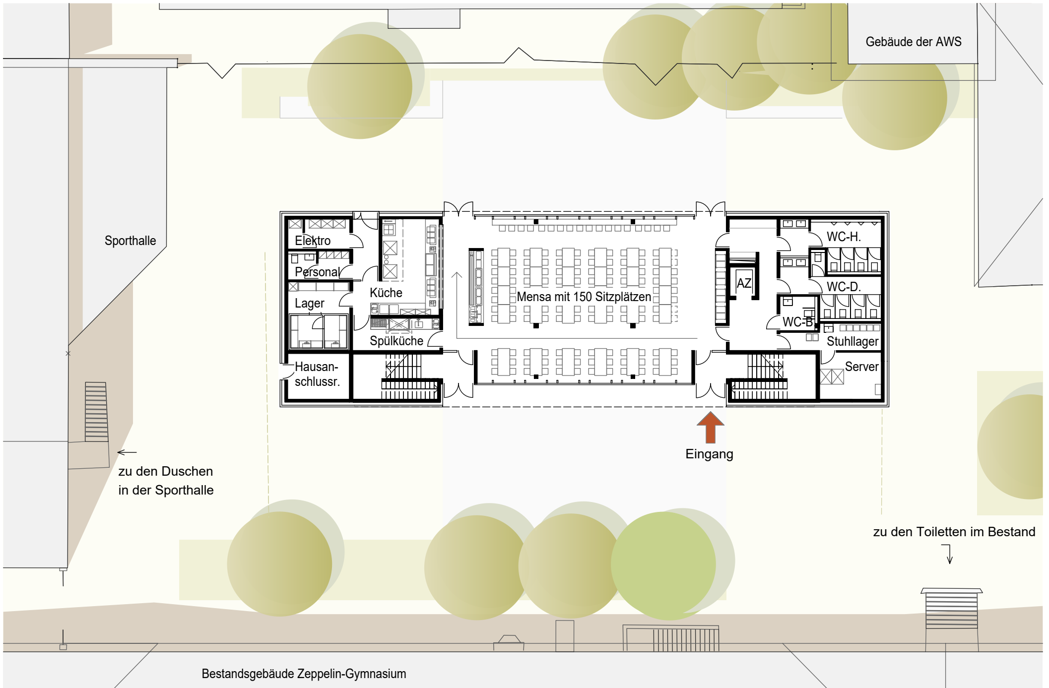
D'Inka Scheible Hoffmann Architekten BDA - Entwurf Mensa und Erweiterung Zeppelin-Gymnasium, Stuttgart Ost - Grundriss EG
