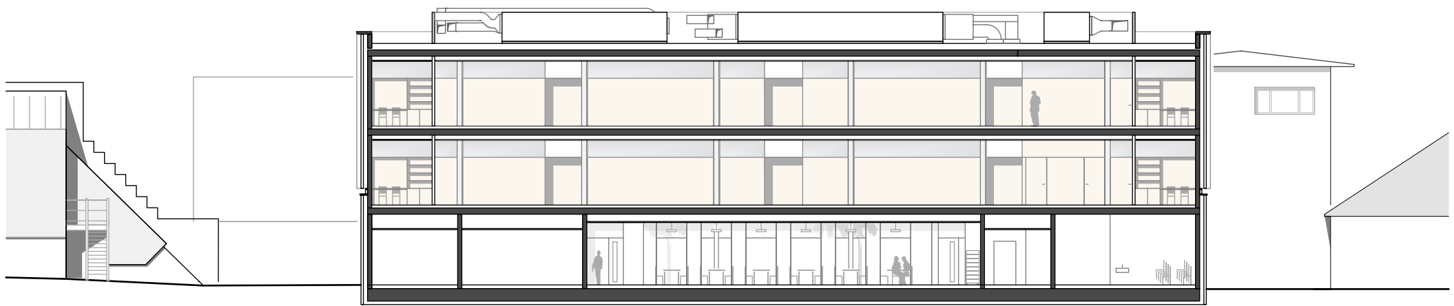
D'Inka Scheible Hoffmann Architekten BDA - Entwurf Mensa und Erweiterung Zeppelin-Gymnasium, Stuttgart Ost - Ansicht Nord-West und Längsschnitt
