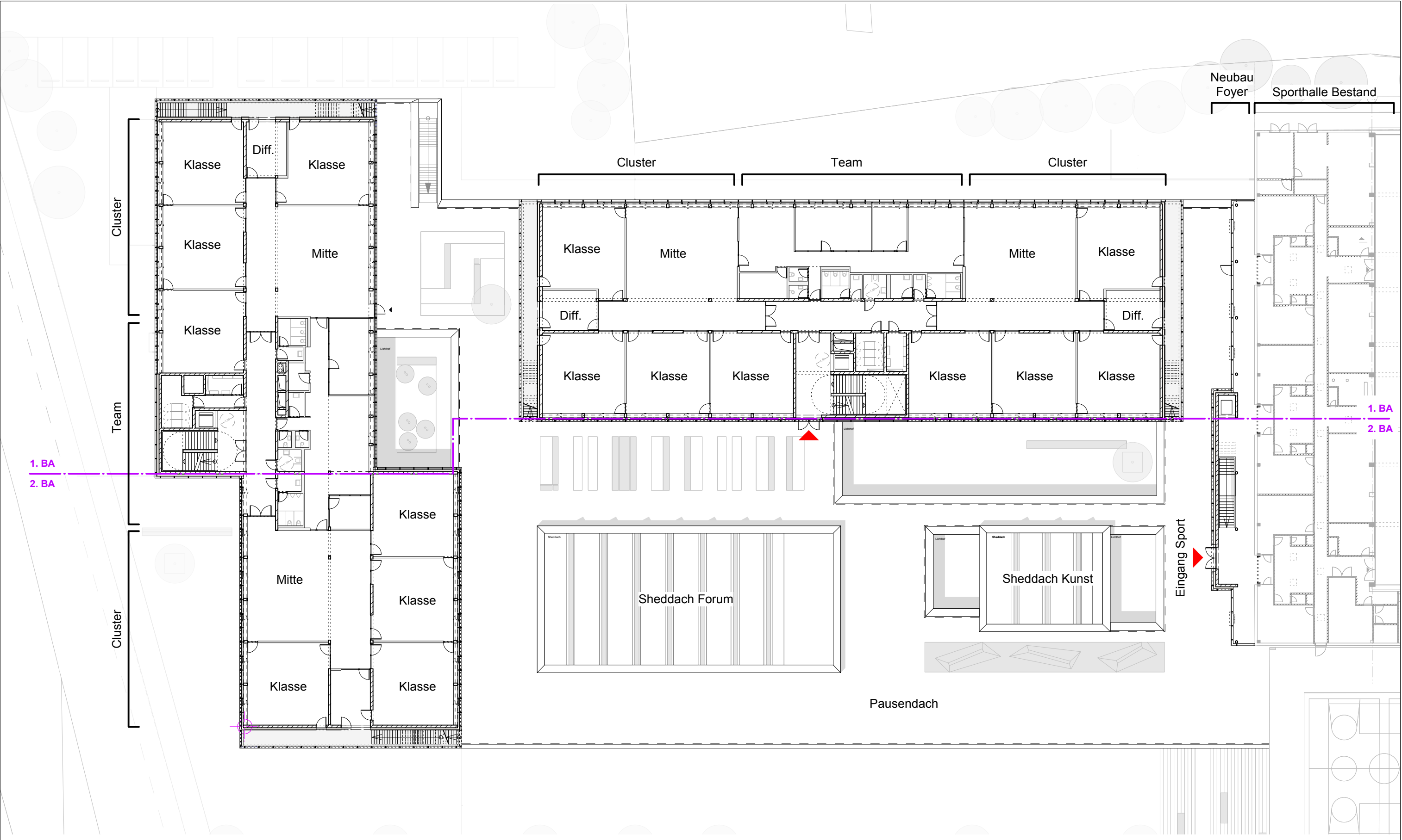
Grundriss 1. Obergeschoss
