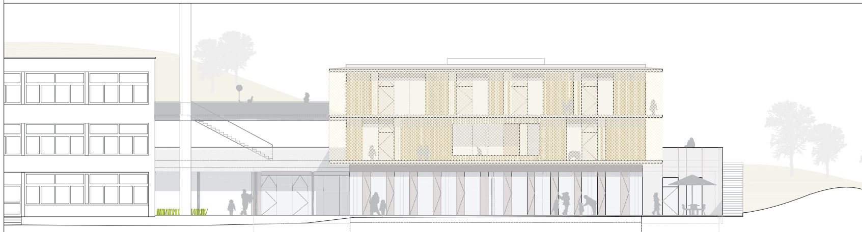
ANSICHT SÜD-OST vom Schulhof
