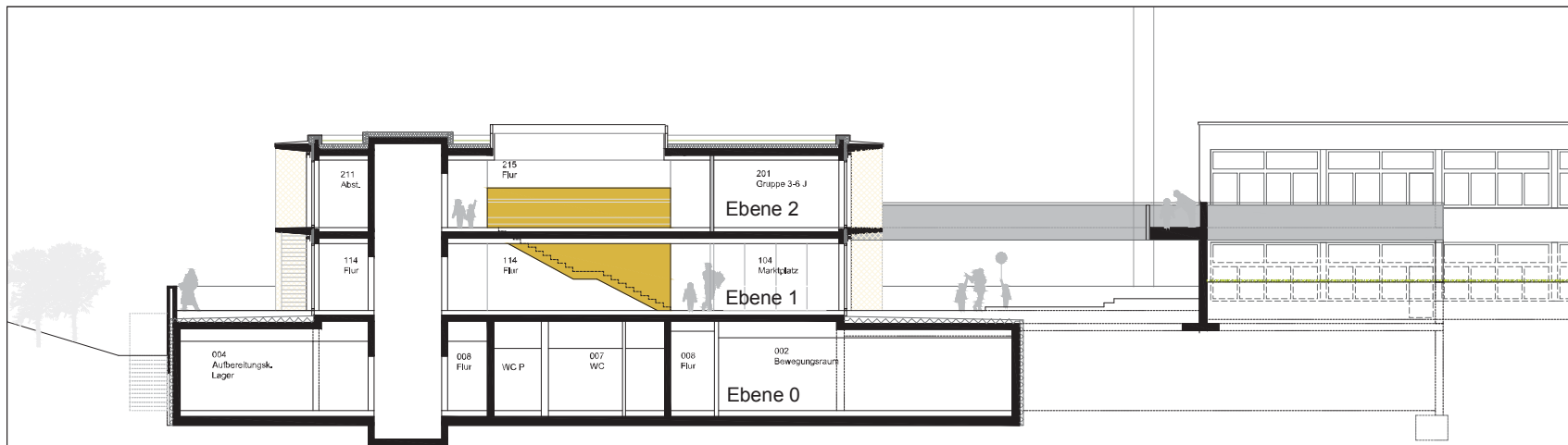
SCHNITT B-B
