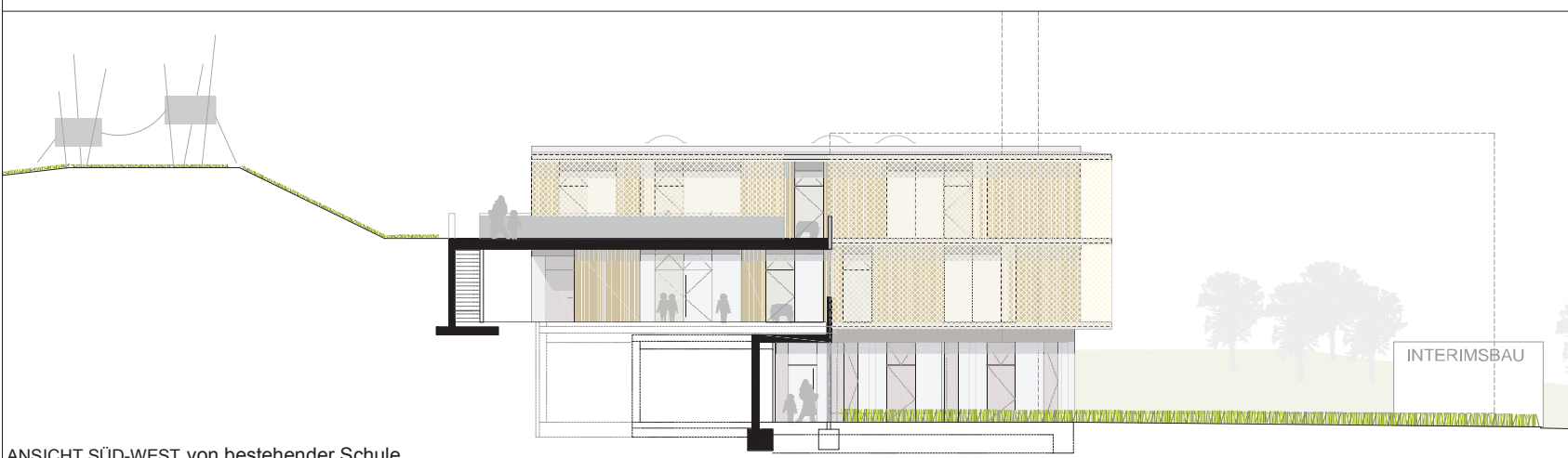
ANSICHT SÜD-WEST von bestehender Schule
