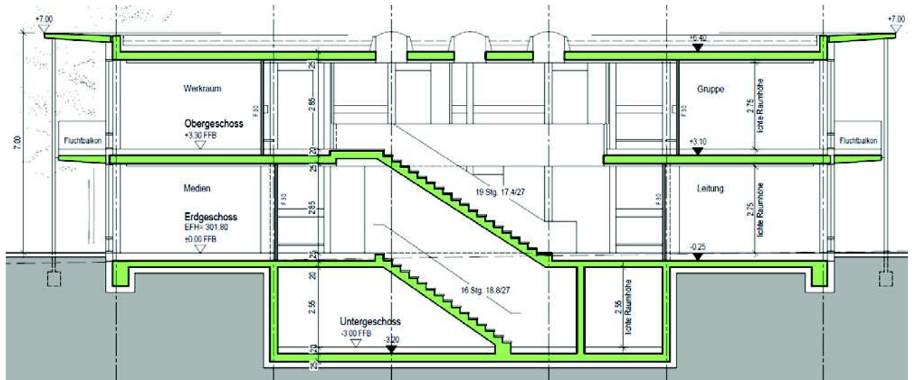
Schnitt A-A
