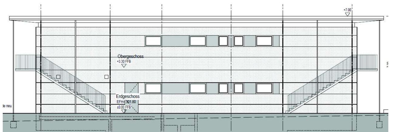
Ansicht Nord
