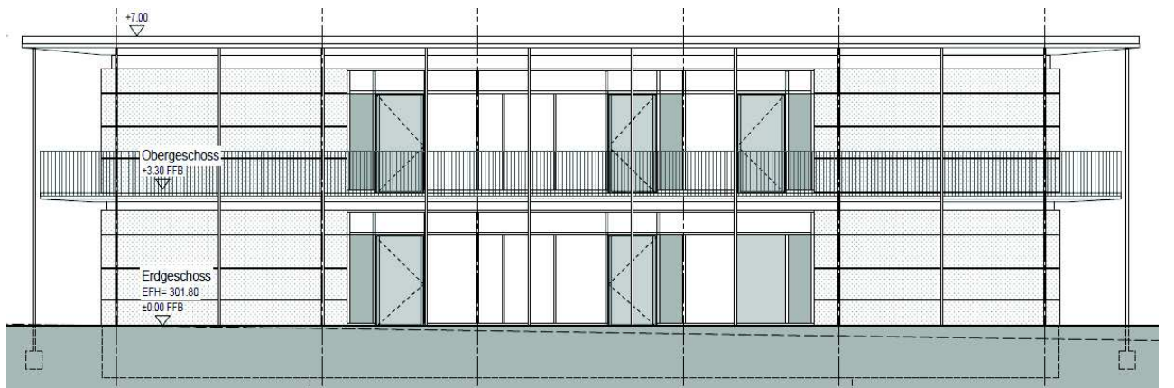
Ansicht Süd
