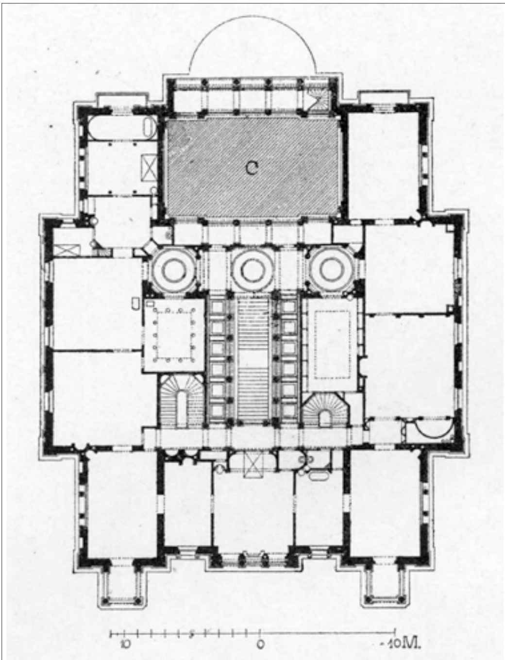
FIGUR 95 Grundriß des oberen Stocks.
