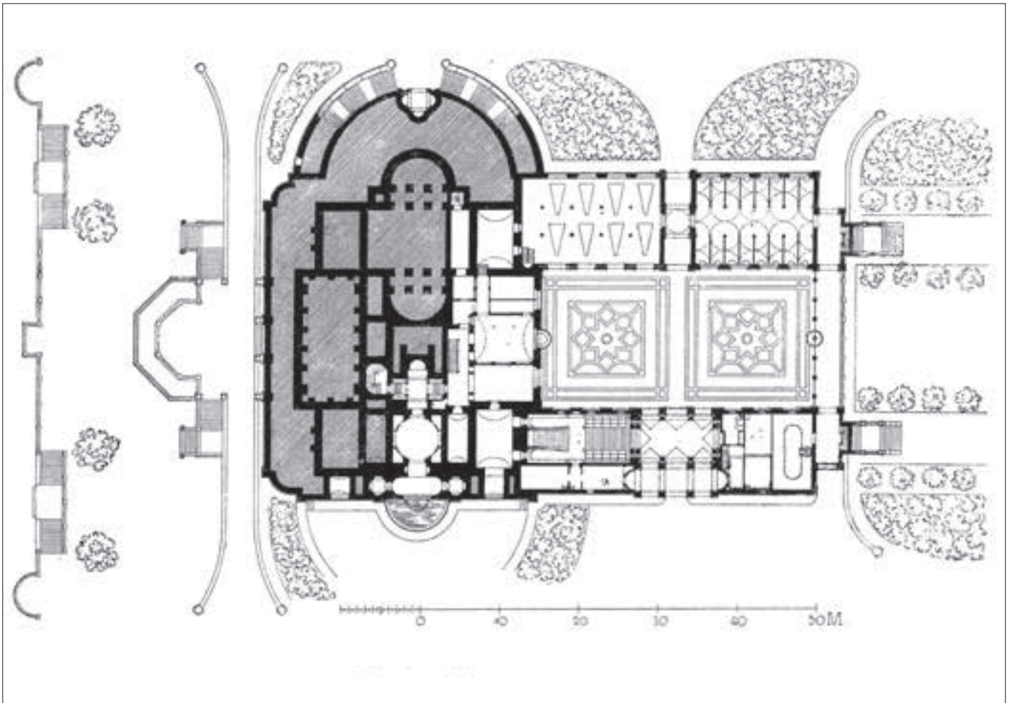
FIGUR 93 Lageplan des Souterrains.
