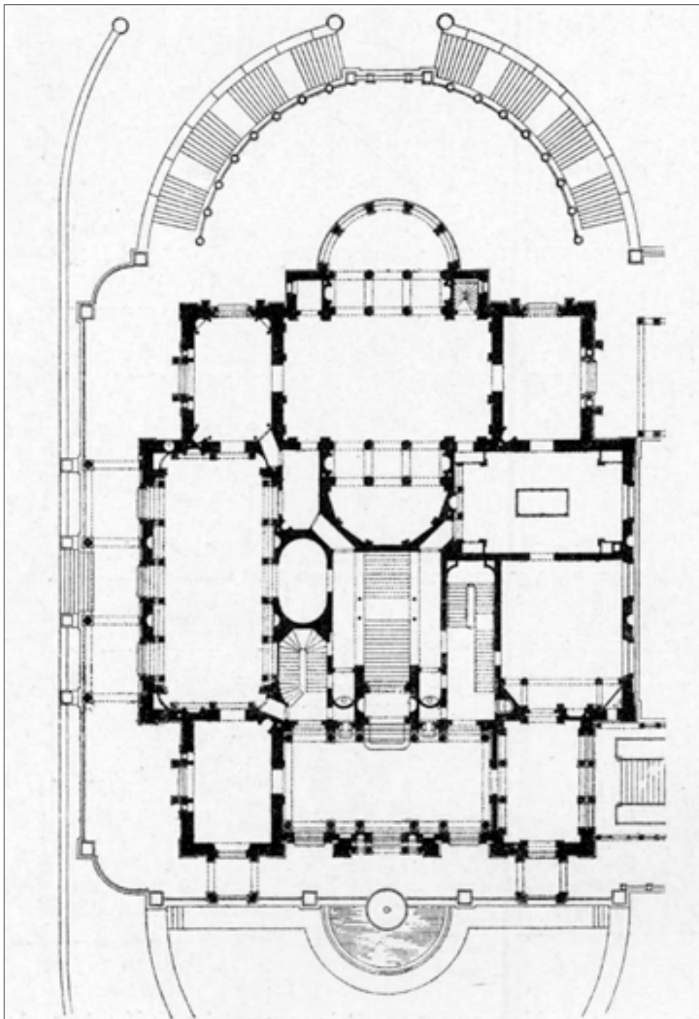
FIGUR 94 Grundriss des unteren Stocks.
